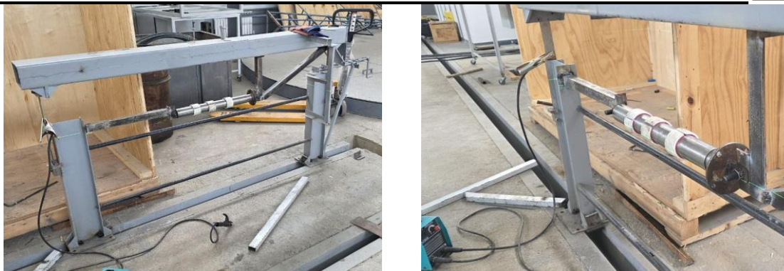
Рис.5. Испытательный стенд и установленное положение демпфера
