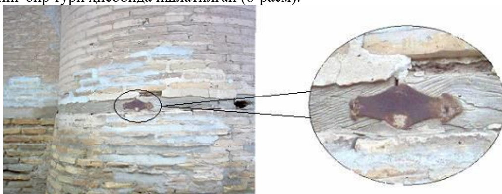
6-расм. Кутлуг Мурад Иноқ мадрасасидаги антисейсмик ёғоч бруслар ва маҳкамловчи метал элементлар (Ичан-Қалъа)
