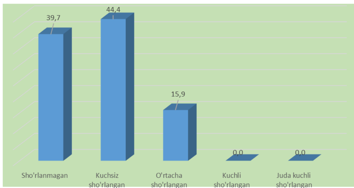
2-rasm. Talishbe massivi sug'oriladigan tuproqlarining sho'rlanganlik darajalari, % hisobida
