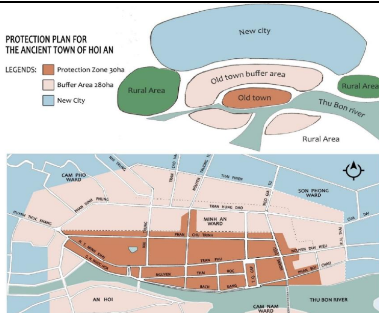
2-rasm. Vetnamning Xoy An qadimiy shahri uchun rayonlashtirish sxemasi va tabiatni muhofaza qilish rejasi.
