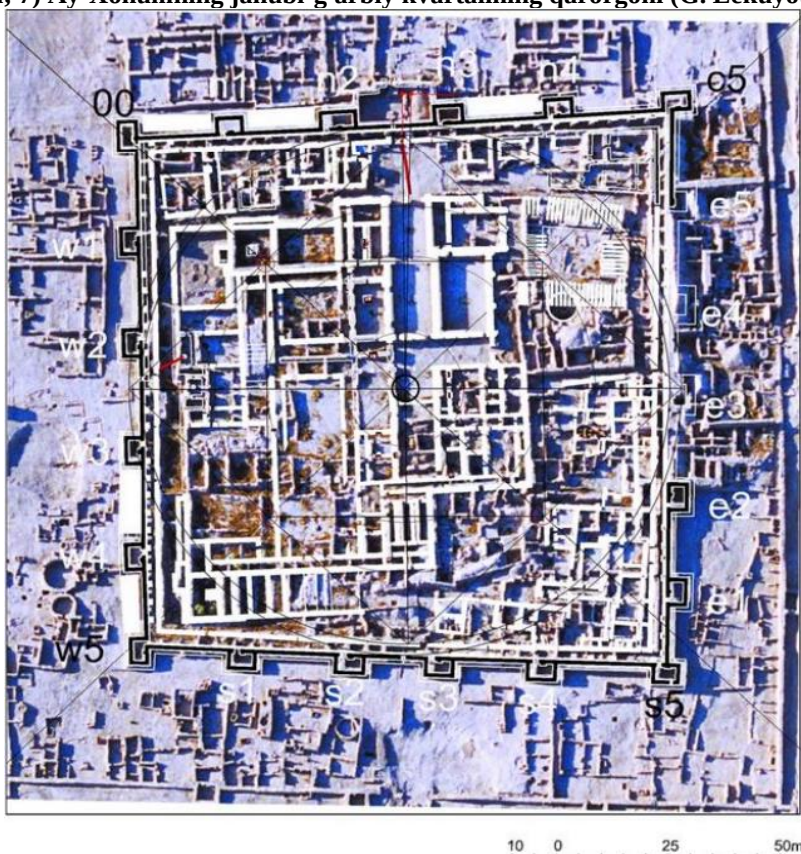
7-rasm. Shimoliy Gongurning aerofotosurati, o'lchovli chizma bilan birgalikda.
