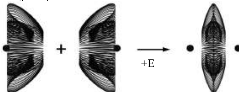
Рис.5. Образование димера пары гамма-нейтронной связи противоположним спином
