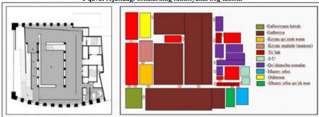
4-rasm. Turkiya Yapi Kredi Madaniy va ma'rifiy, san'at markazi 2-qavat rejasidagi xonalarning funksiyanal bog'lanishi
