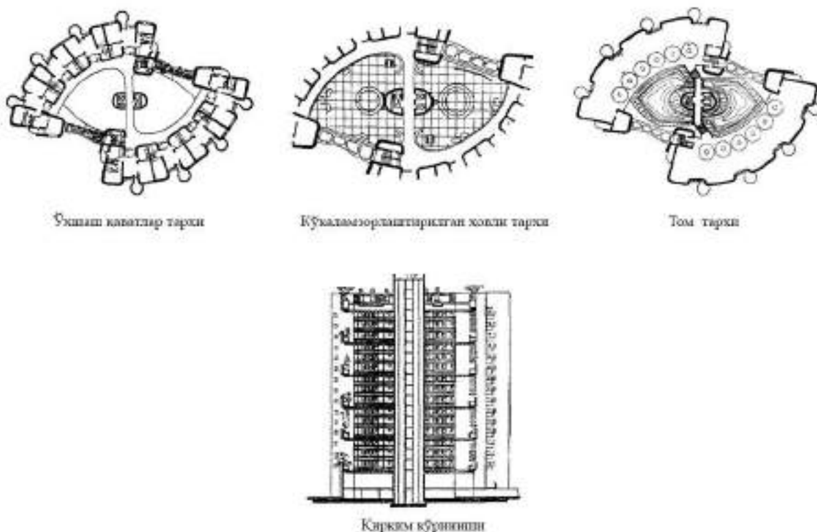
4-расм. 16 қаватли экспериментал турар жой уйи.
