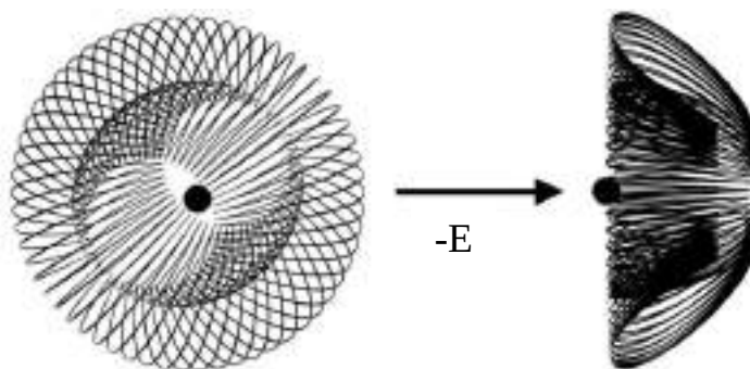
Рис. 4. Торoidalная трансформация нейтронного гамма полусферического орбиталю для связи образования
