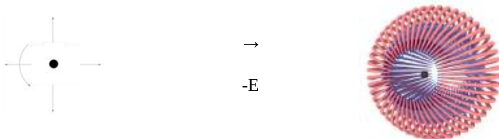
Рис. 8. Схема формирование \beta^+ – ЭМВП вокруг частицы «Asl» с образованием протона
