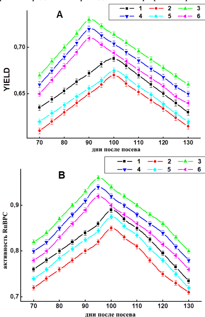
Рис. 1. Зависимость параметров активности фотосинтетического аппарата от фазы вегетации у геннокаутного сорта хлопчатника Порлок-1. А – изменение квантового выхода, В – активность RuBPC. 1 – ноль сегрегант, 2 – Кокер-312, 3 – Т 1-7, 4 – Т 31-10, 5 – АН-Баявут-2, 6 – Порлок-1. По оси абсцисс – дни после посева; по оси ординат – значение квантового выхода (А) или активность ферментов, в мкмоль CO 2 /(мг сырого веса × мин) (В). P ≤ 0,05
