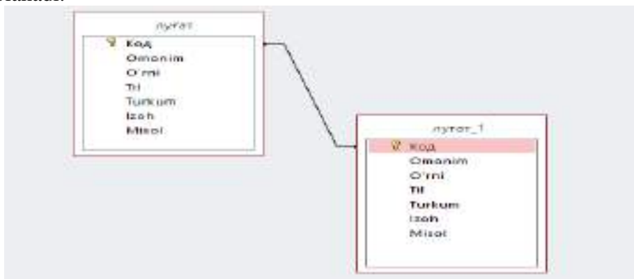
2-rasm. Omonimlar ma'lumotlar bazasining tuzilishi
