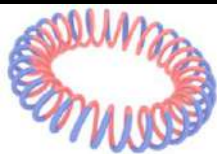
Рис. 1. ЭМВП электрона в свободном состоянии
