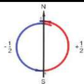
Рис. 2. Срез одного витка спина тороида ЭМВП электрона в магнитном поле в свободном состоянии
