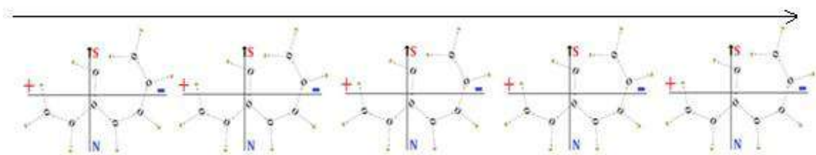
Рис. 14. Генерация электрического тока в атмосферных облачных проводниках
