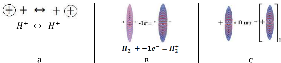
Рис.7. Образование молекулярного иона водорода: а) классический метод, б) метод теории трансформации в) Образование металлического поли ортоводорода
