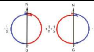
Рис. 3. Тороидный срез спина ЭМВП электронов в магнитном поле в свободном состоянии
