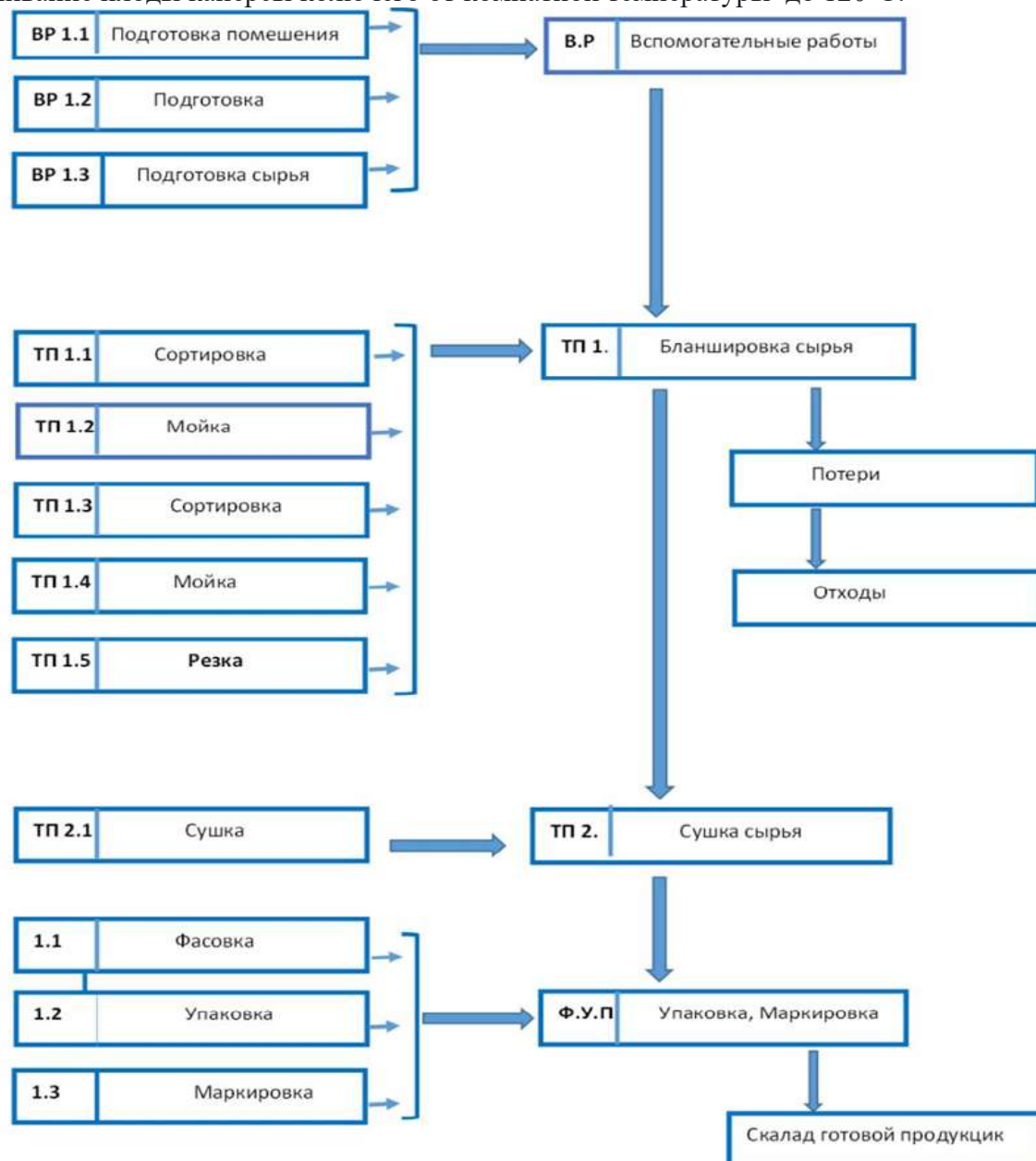
Рис.2. Технологическая схема высушивания плодов лекарственного растения «каперсы колючего» – Capparis spinosa L.
