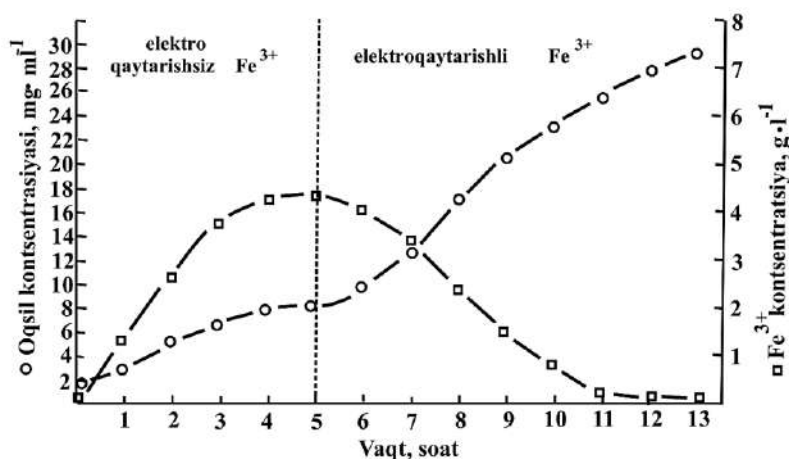
2-rasm. Silverman-Lyudgren K9 muhitida ishqorlovchi bakteriyalar assotsiatsiyasini havo ko'piklantirish bilan elektrokaytarishsiz va elektrokaytarishli uch valentli temir ishtirokida yetishtirish
