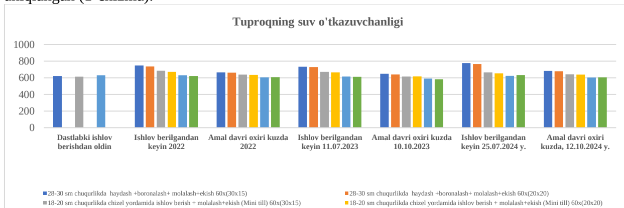
1-chizma. Yerga turli usulda ishlov berib marjumak va rijik parvarishlanganda tuproqning suv o'tkazuvchanligi, m 3 /ga
