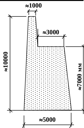
1-расм. Дешон Қалъа деворининг ва қирқимининг кўриниши
