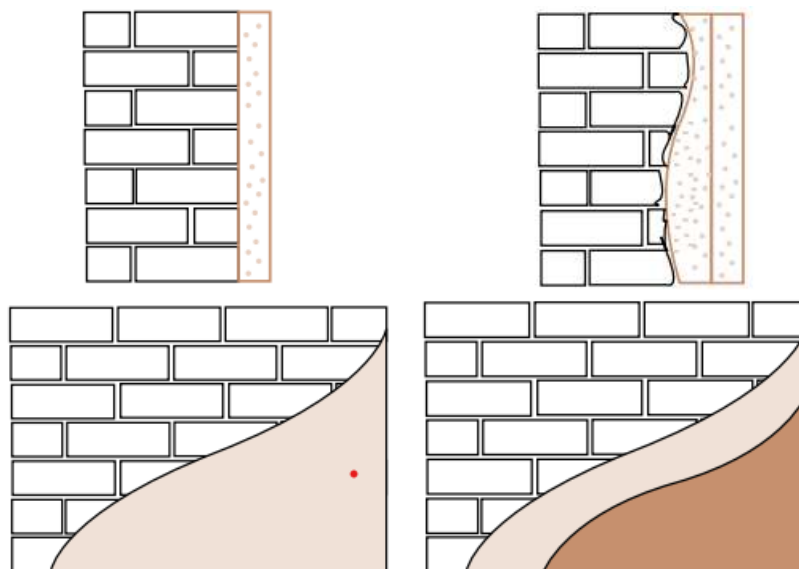
5-расм. Бир қатлам қилиб сувоқ қилинганда.
