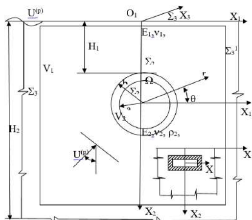
Рис. 1 Расчетная схема
