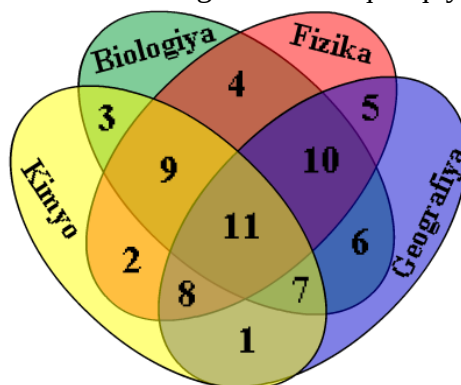
1-rasm. Tabiiy fanlarning o'zaro aloqadorligi bo'yicha Venn diagrammasi
