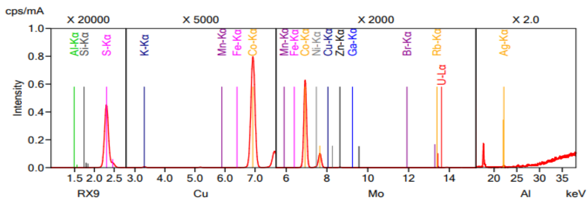
1 – расм. [\text{Co}(\text{L})_2(\text{H}_2\text{O})_2] нинг рентгенофлуоресцент спектри
