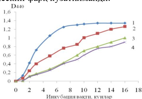
1-расм. Амарант уруғи оксилларидан нейтраза ферменти ёрдамида олинган пептидларнинг (+)-катехинни оксидланиш жараёнига таъсири.
