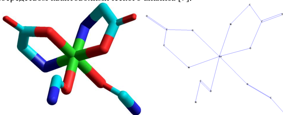
Рис.1. Пространственное строение молекулы [Cu(Gl-H) 2 2FA]
