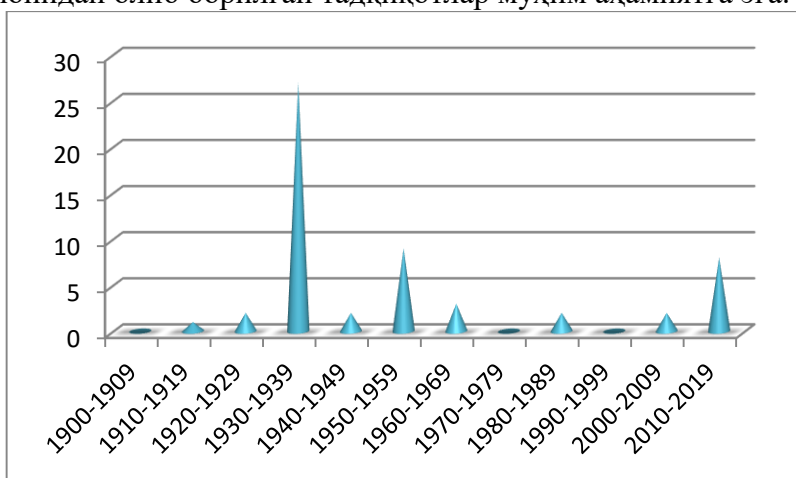
2-расм. TASH фондидаги Tulipa L. турлари гербарий намуналарининг йиллар бўйича тақсимланиши
