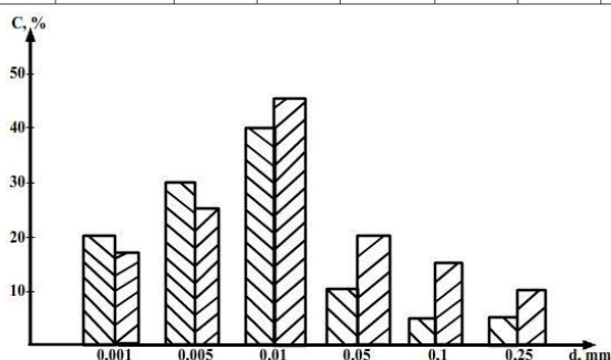
1-расм. Базиргон ва Туямўйин конлари гилсимон хом ашёларининг гранулометрик таркиби
