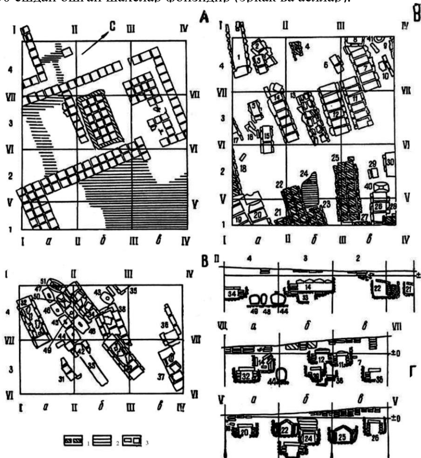
1-расм. Миздахкон қабристони. №2, 3, 4, 6, 10, 18, 29 -сонли болалар қабрлари Қазиш ишлари - 1. Режа: А – қабр даражаси бўйича; В – 1-2 қатлам даражасида; В – 2-3 қатлам даражасида; Г – кесмалар; 1-пишган ғишт ва тош; 2-лой блоклар; 3-хом ғишт
