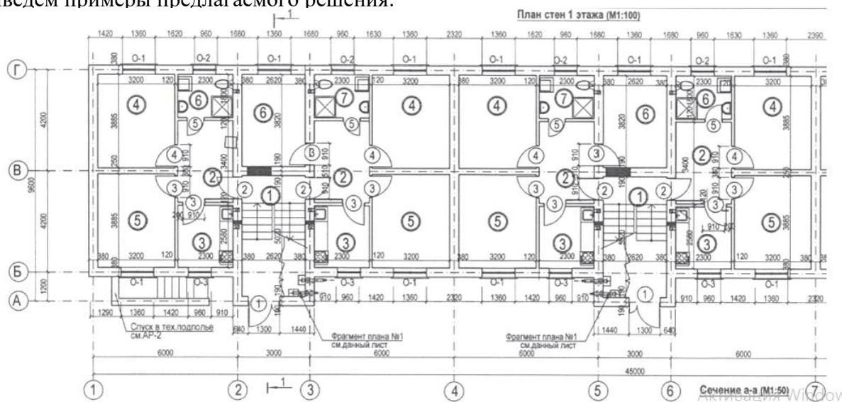
Рис.2. Фрагмент плана стен 1-го этажа 4-х этажного 24-квартирного жилого дома.
