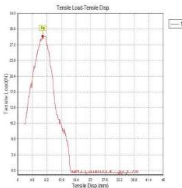
Рис.3. График прочности на растяжение.
