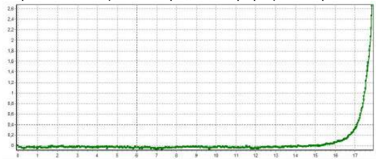
Рис. 9. График испытания полученной пасты на сжатие.
